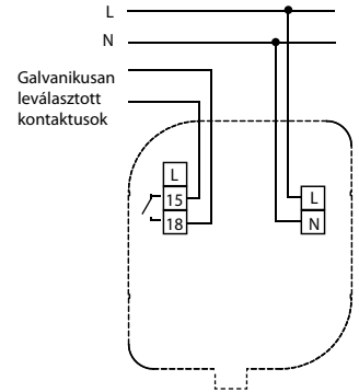
4 - vezetékes csatlakozás
