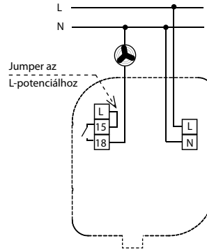
3 - vezetékes csatlakozás
